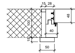
5 Jamb Detail 1 : 5
