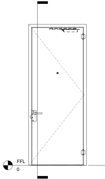
2 Door Elevation 1 : 20
