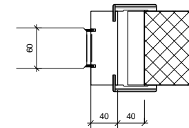
5 Jamb Detail 1 : 5
