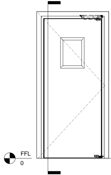
2 Door Elevation 1 : 20
