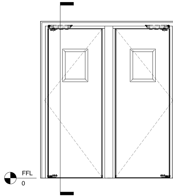
2 Door Elevation 1 : 20
